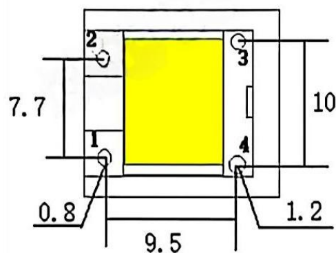
底视图
