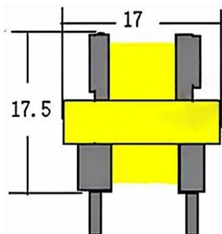
正视图
