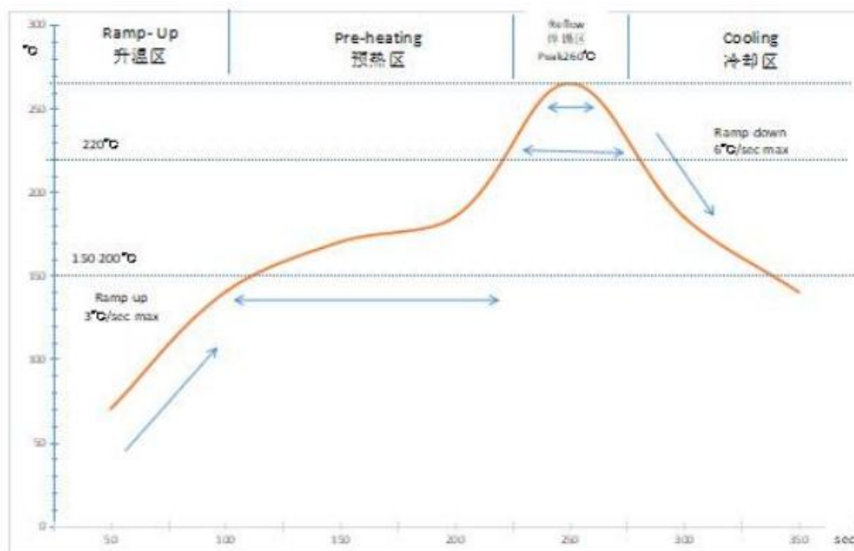
Lead-Free(LF)标准温度分析范围
