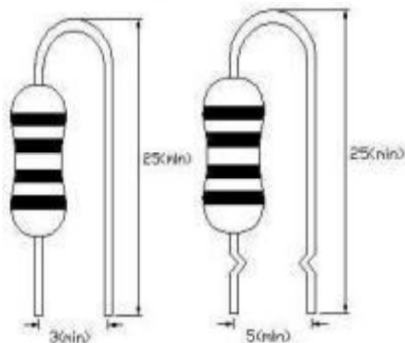
弯脚成型 ( V type ) 弯脚 K 型 ( VK type )
