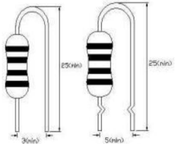
弯脚成型 ( V type ) 弯脚 K 型 ( VK type )
